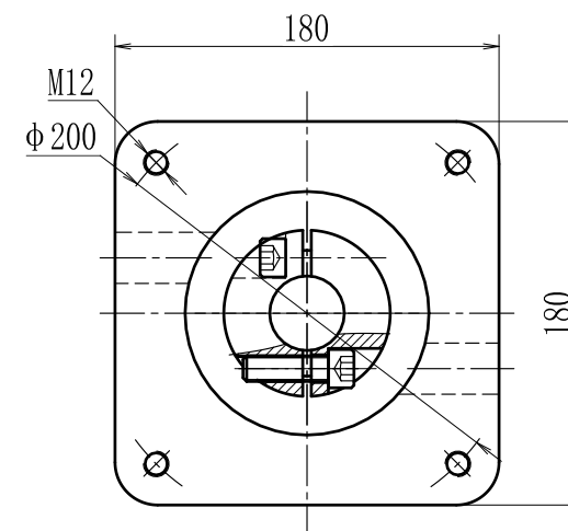
输入轴
